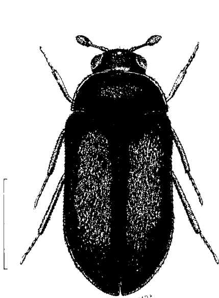
Globicornis nigripes
