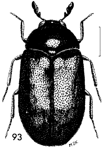
Ctesias serra
