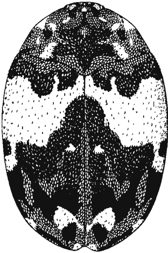
pimpinellae
