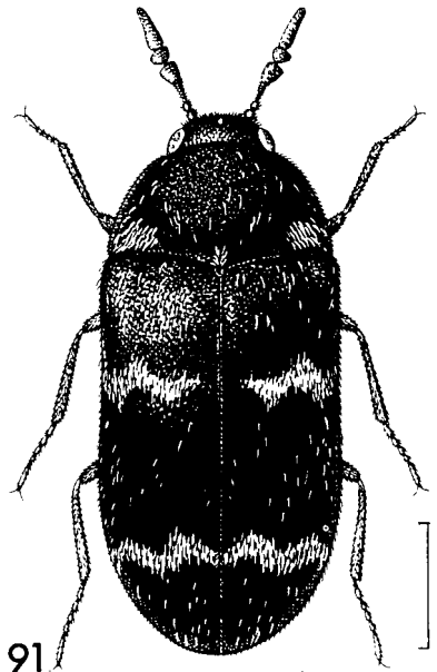
Megatoma undata
