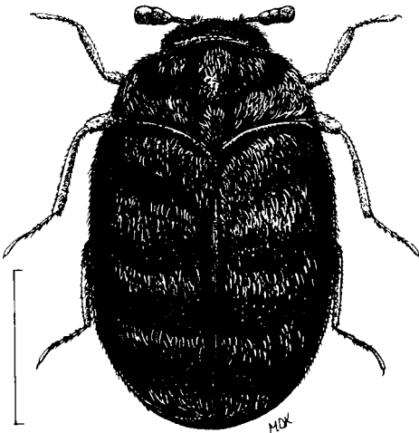
Anthrenocerus australis
